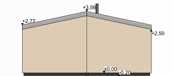
RÜCKFASSADE
